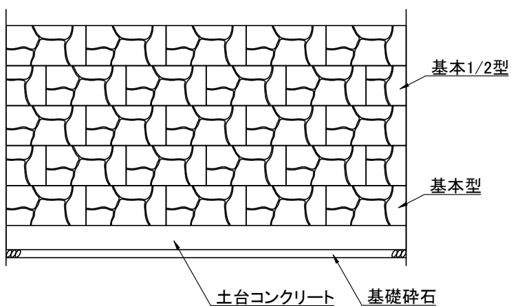
展開図
