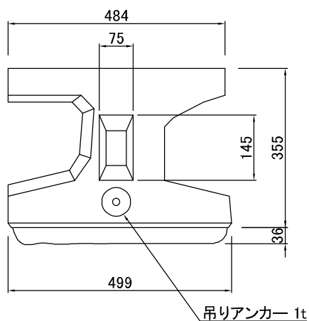
規格表
