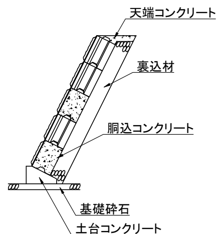
断面図
