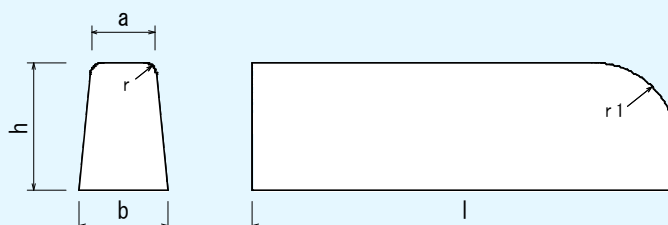
歩道用境界ブロック (コーナー)
