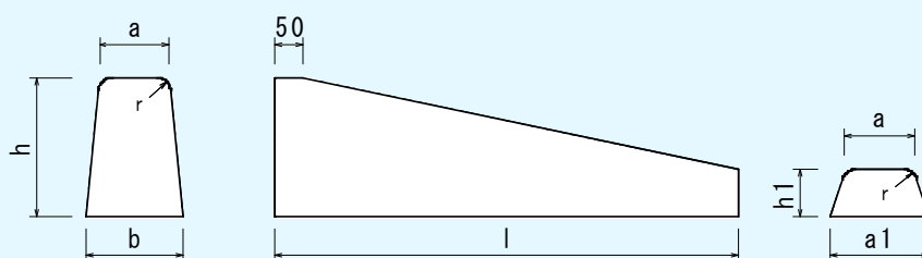
歩道用境界ブロック (三 角 部)
