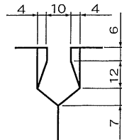
目地部詳細図
