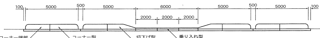
デリネーター用詳細図
