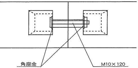
連結部詳細図
