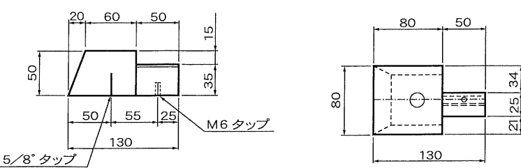
連結部詳細図
