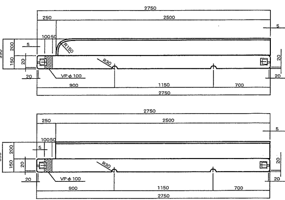
目地部詳細図
